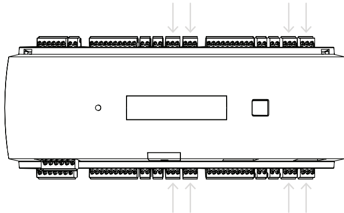
Рис. 4.17: Расположение разъемов релейных выходов
