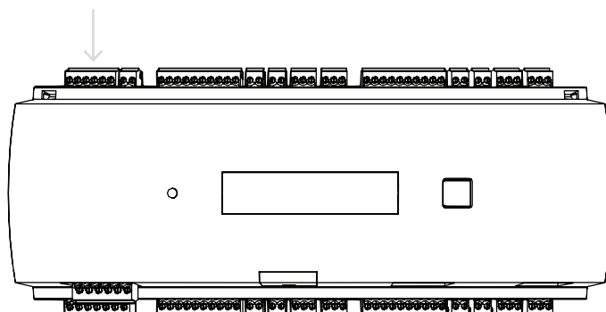
Рис. 4.14: Расположение шины модуля расширений RS-485
