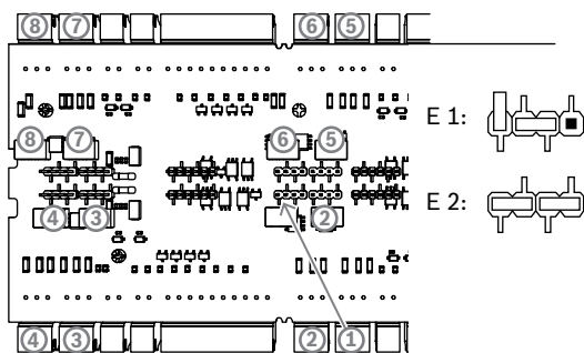
Рис. 4.20: Расположение перемычек релейных выходов (тыльная сторона)
