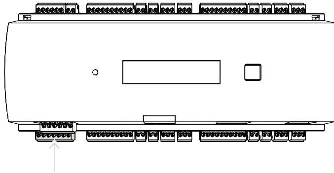
Рис. 4.7: Местоположение разъема источника питания
