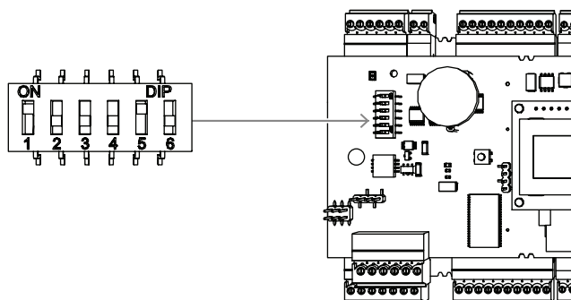
Рис. 4.13: Расположение селектора для настройки параметров главного компьютера и состояние при поставке
