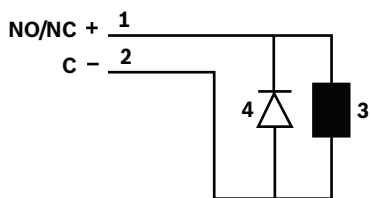
Рис. 4.19: Схема восстановительных диодов
