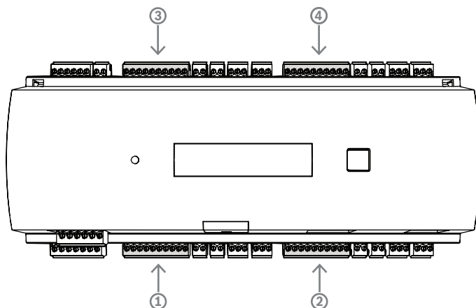
Рис. 4.16: Расположение интерфейса (порта) Wiegand для считывателей
