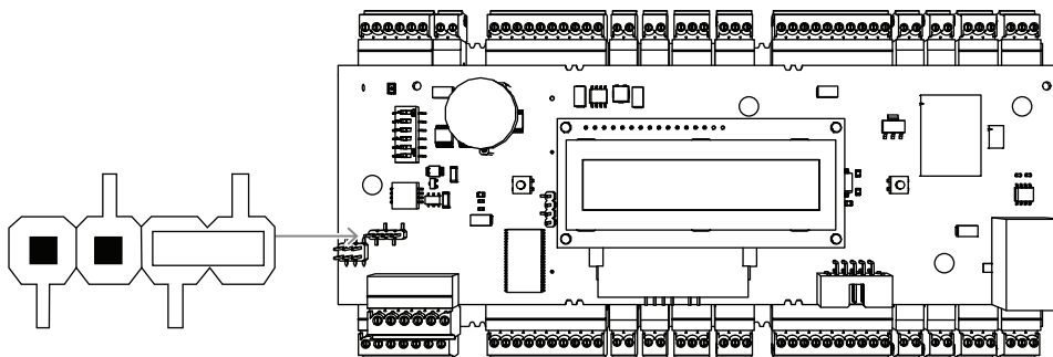
Рис. 4.11: Настройка переключек для двухпроводных подключений RS-485
