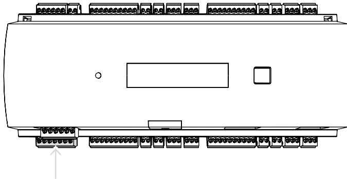
Figura 4.7: Posizione del connettore di alimentazione
