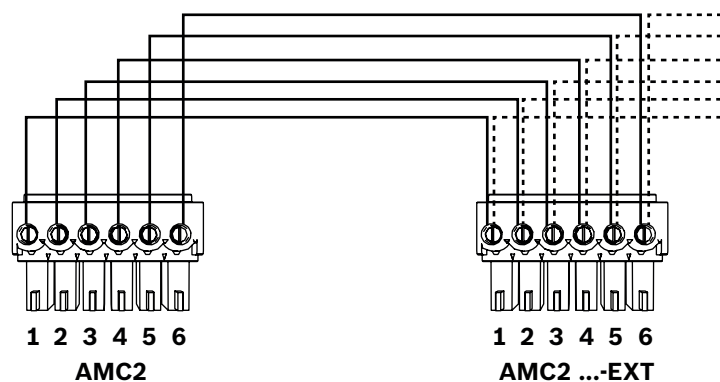
Figura 4.15: Connessione di un modulo di estensione a un'unità di controllo
