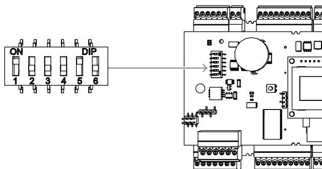
Figura 4.13: Posizione del selettore per impostazioni host e stato di recapito
