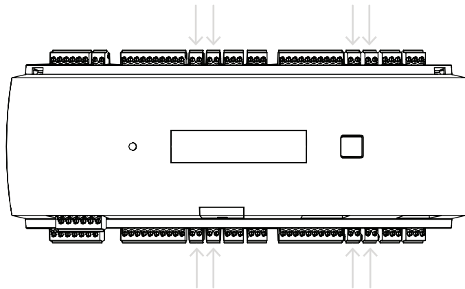
Figura 4.21: Posizione dei connettori di ingresso analogici
