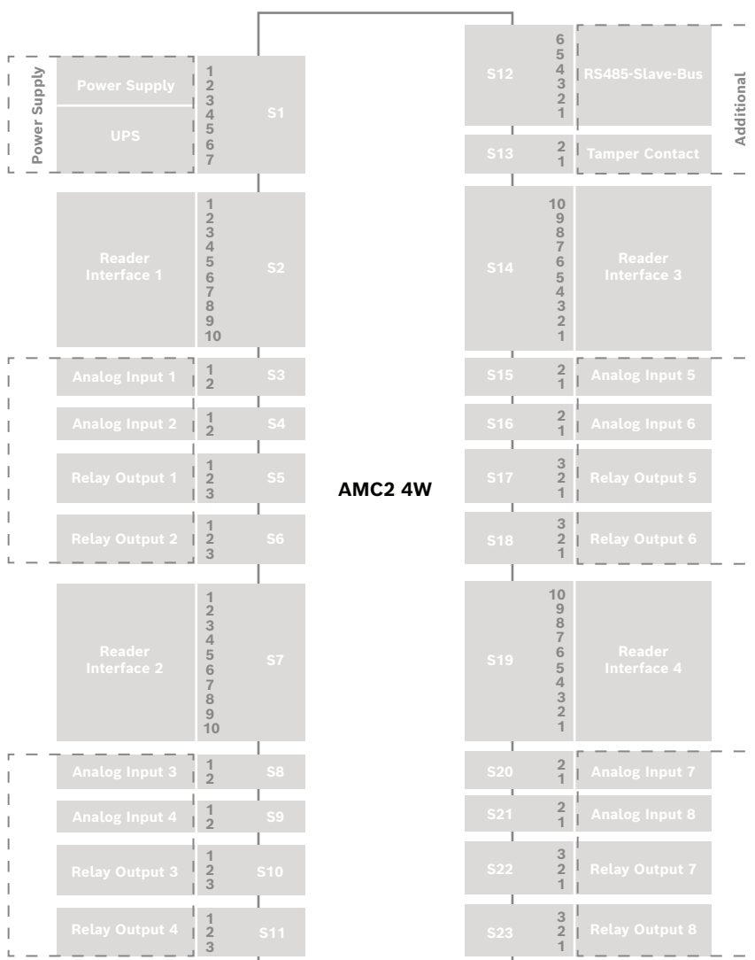
Figura 11.3: Blocchi connettore dell'AMC2-4W
