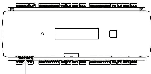
Figura 4.10: Interfaccia host RS-485
