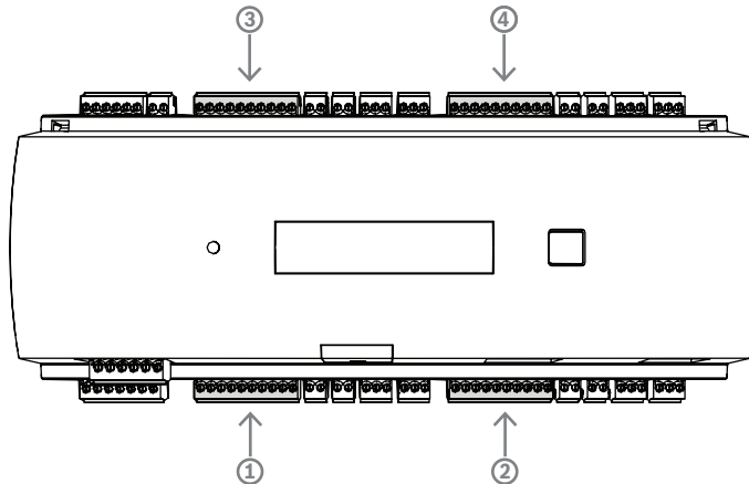
Figura 4.16: Posizione dell'interfaccia Wiegand (porta) per i lettori
